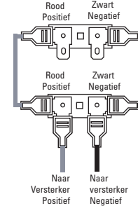
Afbeelding 2. Twee woofers parallel aansluiten op de versterker (2 ohm).
