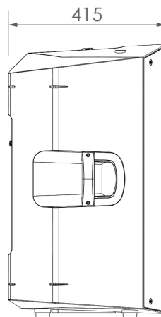
Vista lateral
