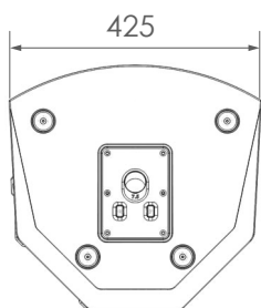
Vista inferior
