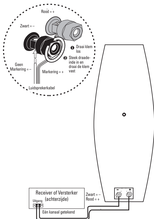
Afbeelding 3. Het blokschema geeft de juiste polariteit aan voor één kanaal van een home theater systeem.
